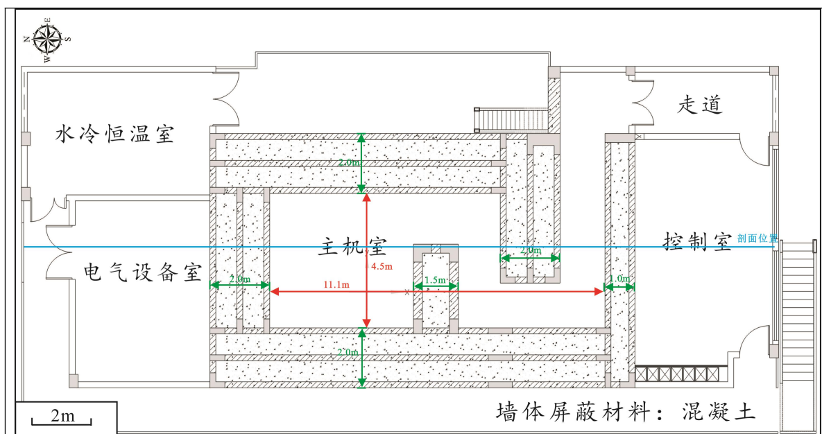
图 1-6 二层主机室平面布局图
