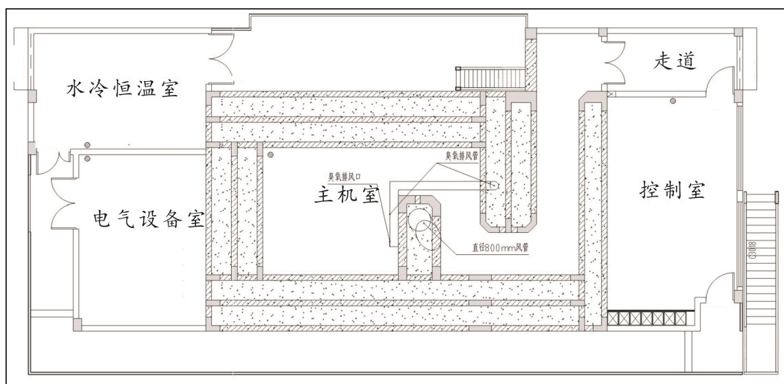
图 10-7 排风管道示意图 2
