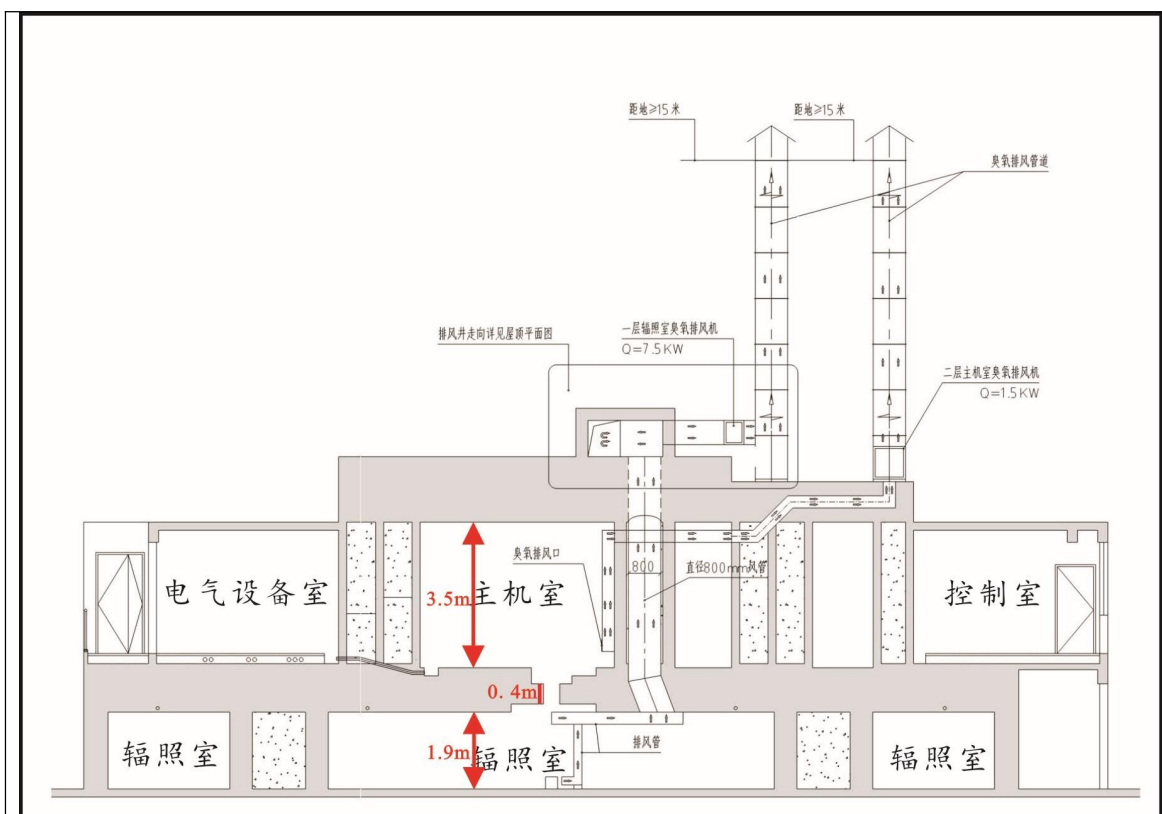
图 10-6 排风管道示意图 1
