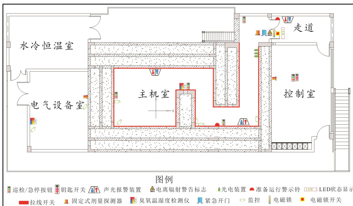
图 10-3 一层辐照室辐射安全设施图
