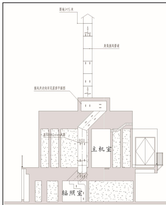
图 10-8 排风管道示意图 3
