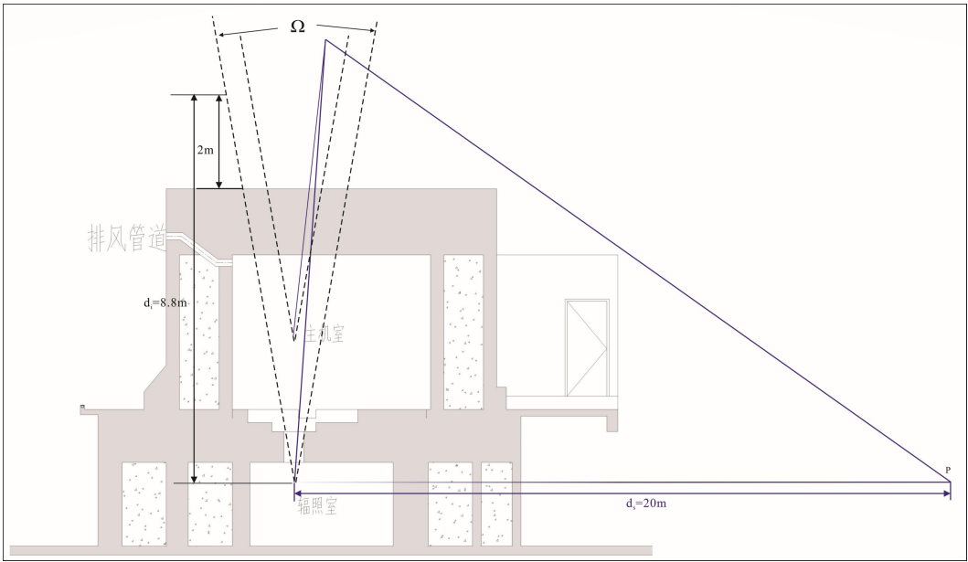
图 11-6 天空反散射示意图
