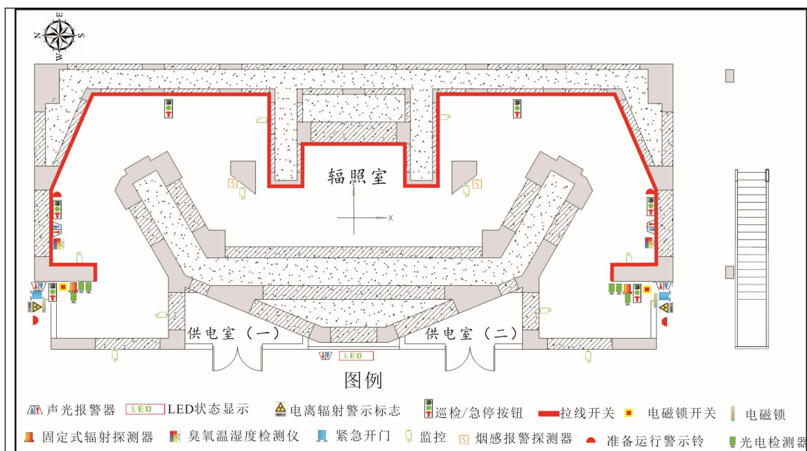
图 10-3 一层辐照室辐射安全设施图
