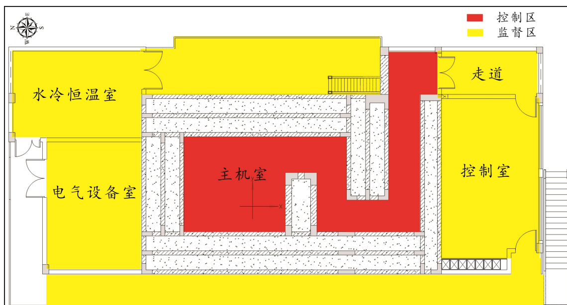
图 10-2 辐照机房二层分区示意图
