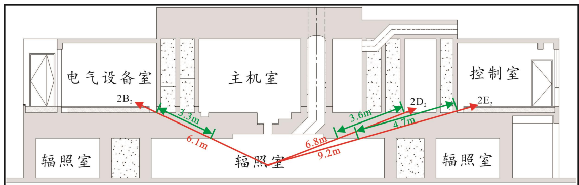
图 11-2 二层主机室四周各关注点位分布图
