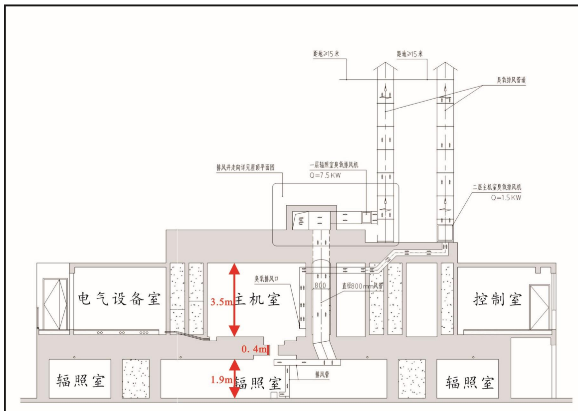
图 1-7 剖面图
