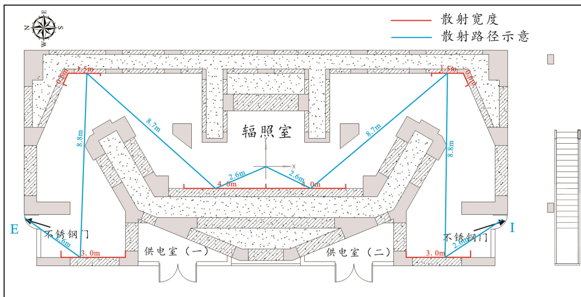
图 11-5 一层辐照室散射路径示意图
