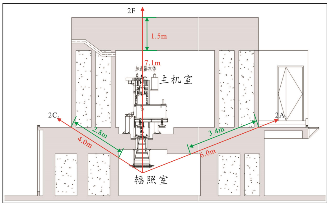
图 11-3 辐照机房剖面图 1 关注点位分布图
