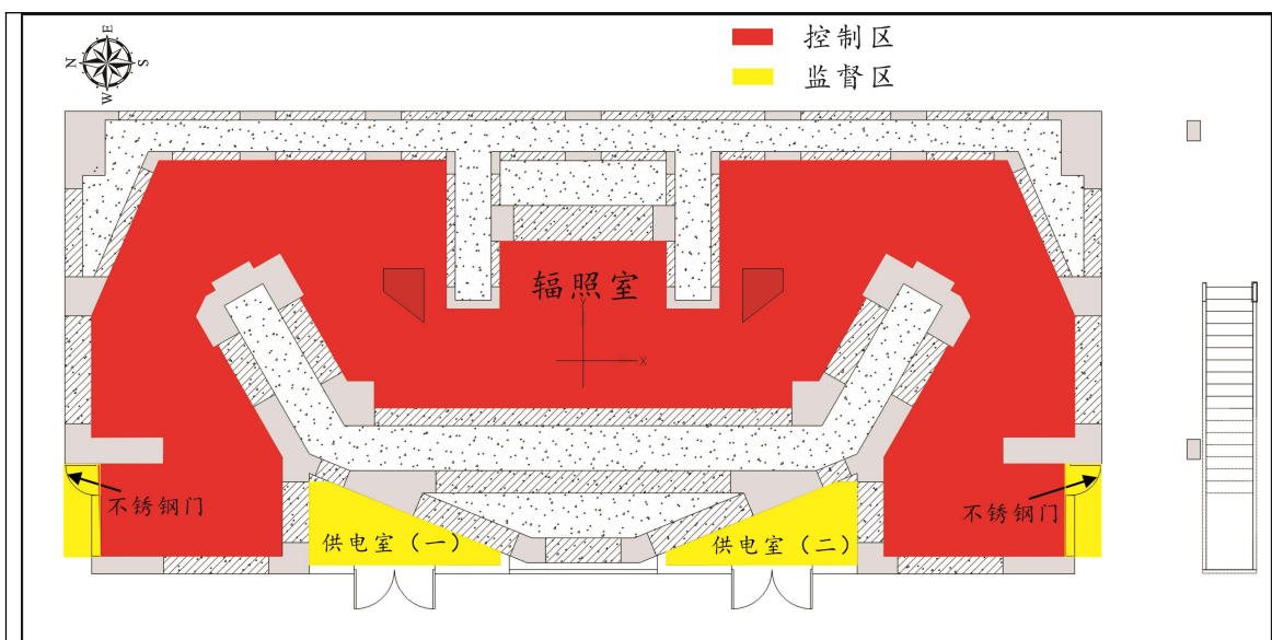
图 10-1 辐照机房一层分区示意图
