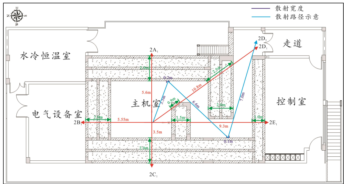
图 11-2 二层主机室四周各关注点位分布图
