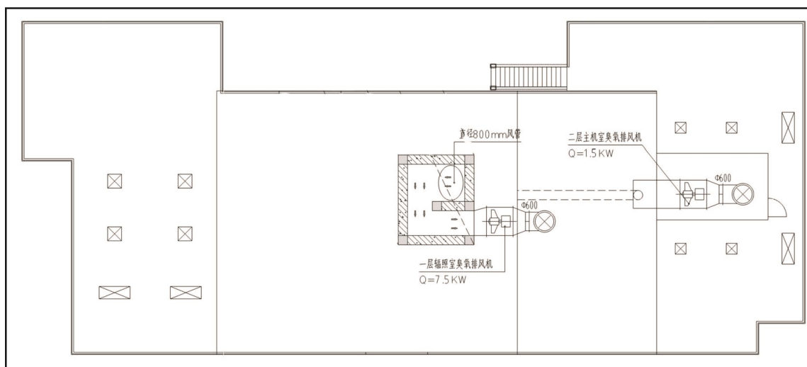
图 10-9 屋顶排风机位置示意图
