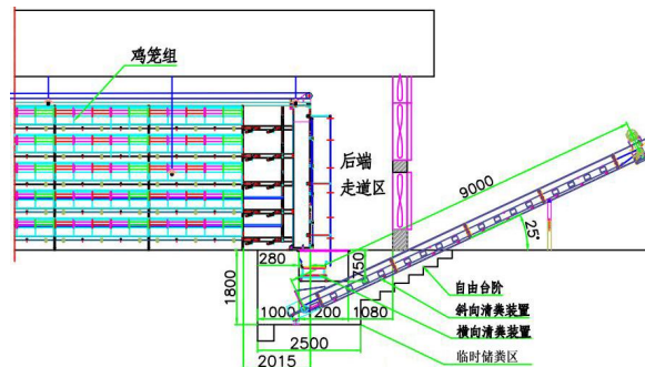
图 3.2-2 本项目清粪工艺示意图
