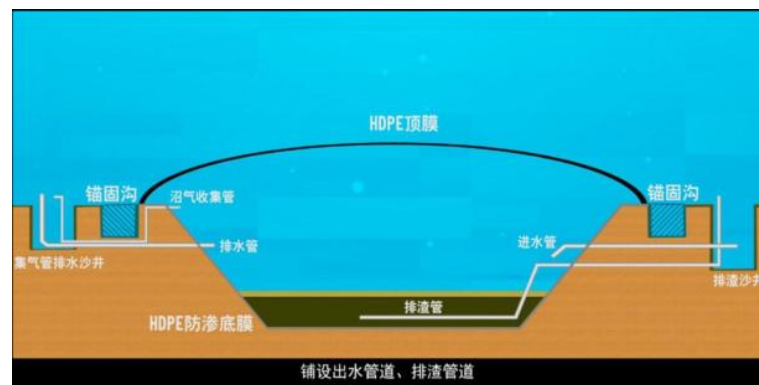
图 3.2-3 黑膜沼气池结构示意图
