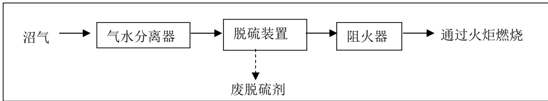
图 3.2-4 沼气净化工艺流程图
