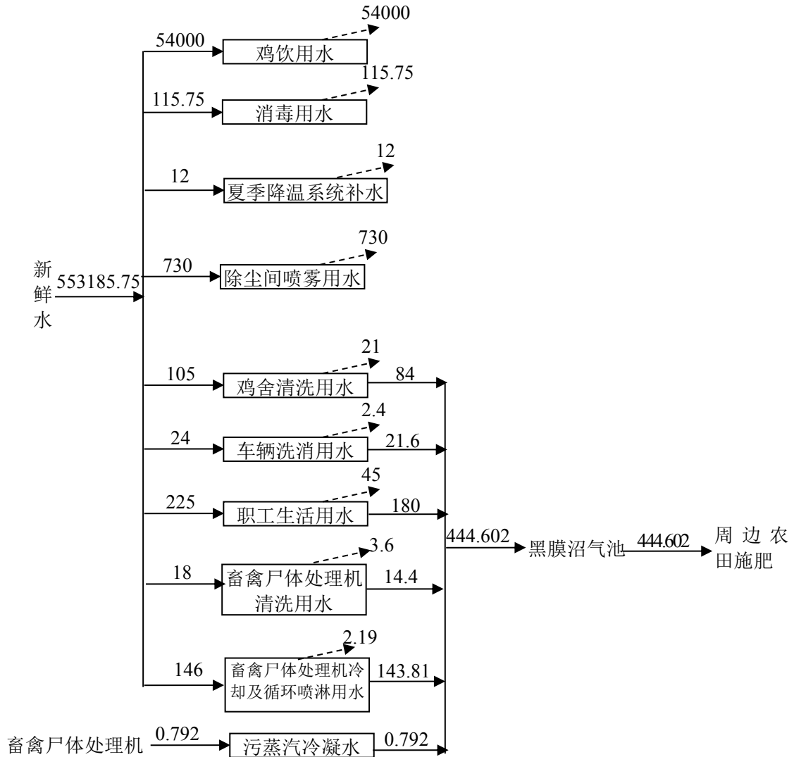
图 3.2-6 本项目水平衡图（单位：m³/a）
