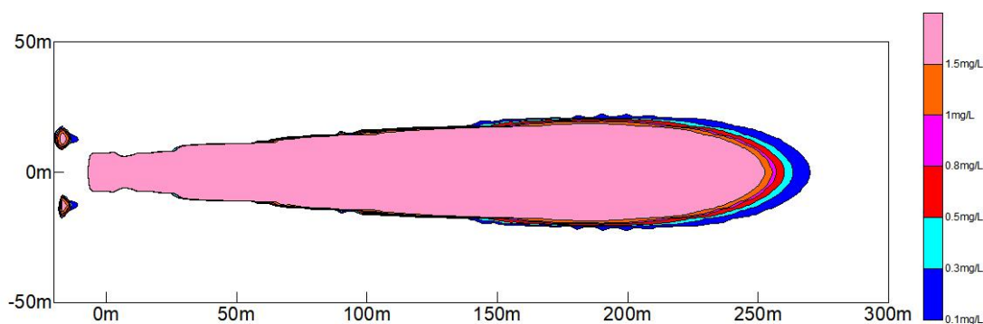
(3) \text{NH}_3\text{-N} 泄漏 1000 天
