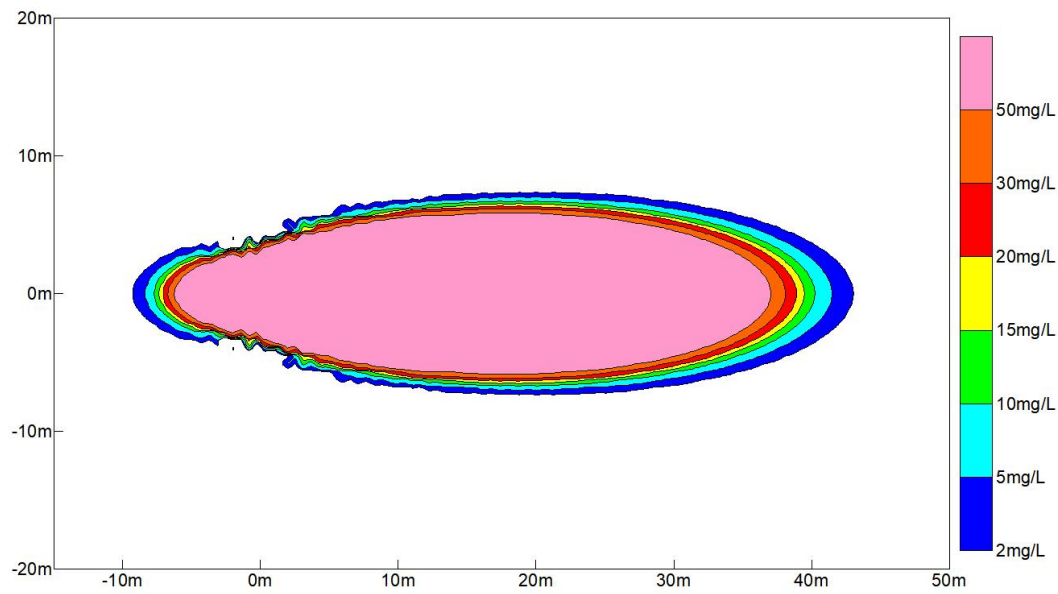
(2) COD 泄漏 100 天
