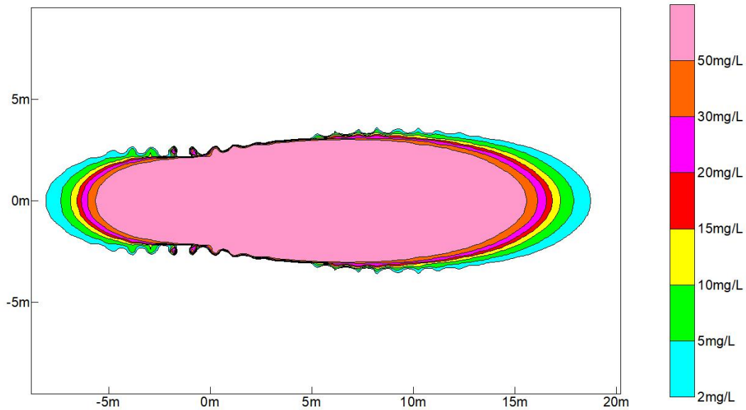
(1) COD 泄漏 30 天
