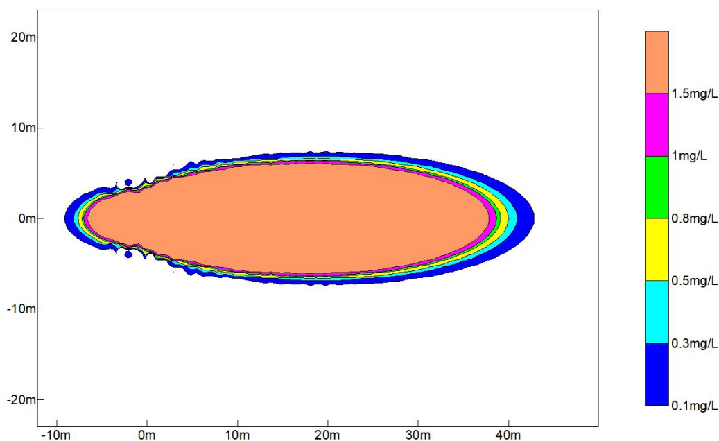
(2) \text{NH}_3\text{-N} 泄漏 100 天
