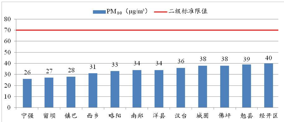
图5 2024年4月各县(区)PM 10 浓度及达标情况
