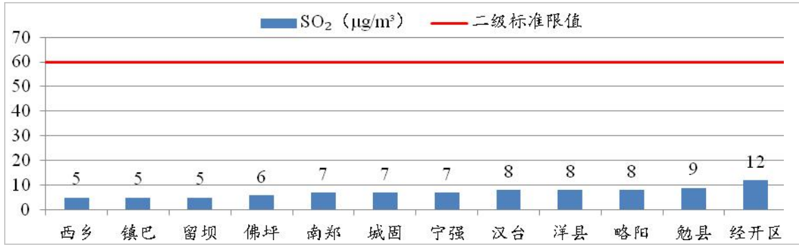
图 17 2024 年 1~4 月各县（区）SO 2 浓度及达标情况
