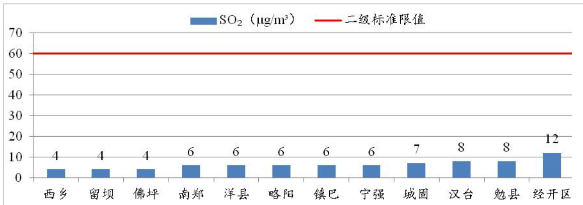
图7 2024年4月各县(区)SO 2 浓度及达标情况
