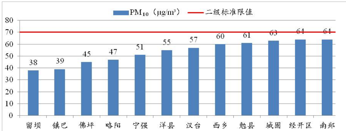
图 15 2024 年 1~4 月各县（区）PM 10 浓度及达标情况
