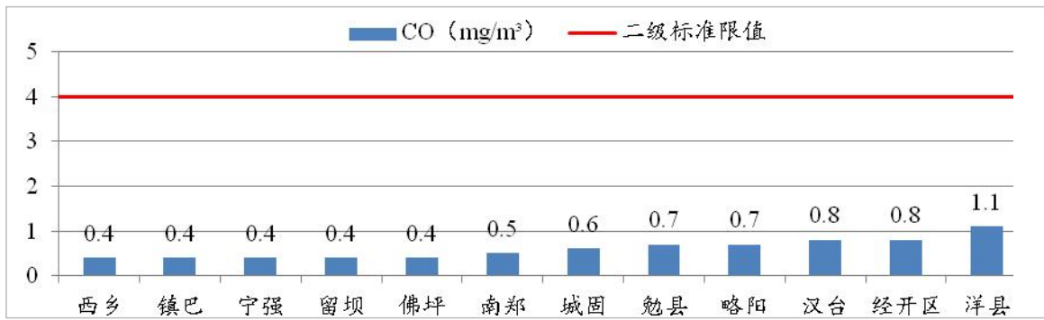
图9 2024年4月各县(区)CO浓度及达标情况
