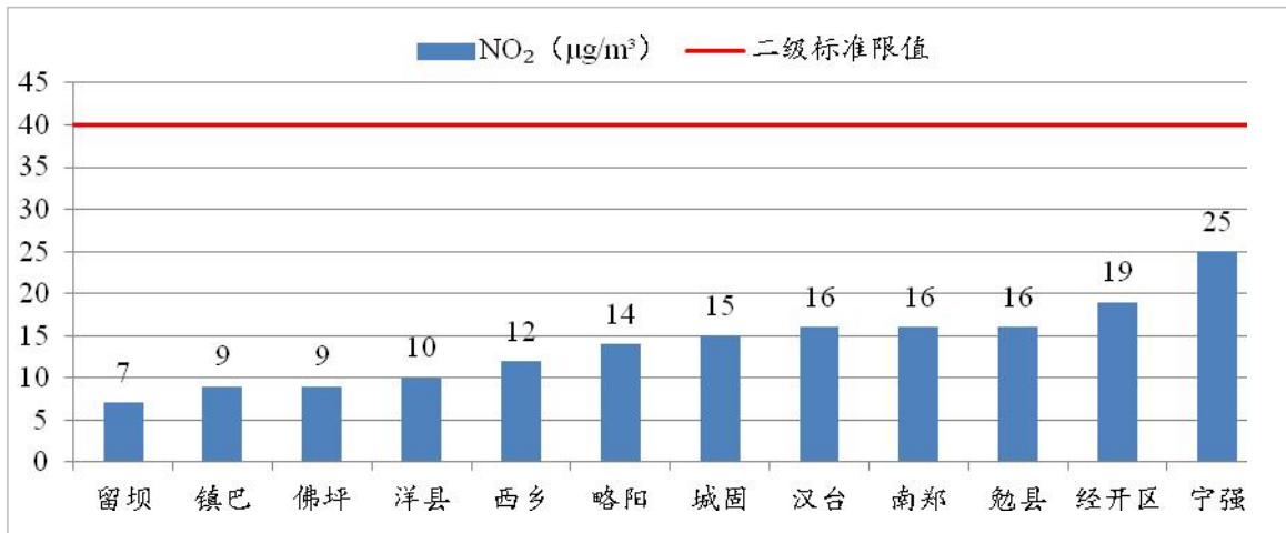
图8 2024年4月各县(区)NO 2 浓度及达标情况
