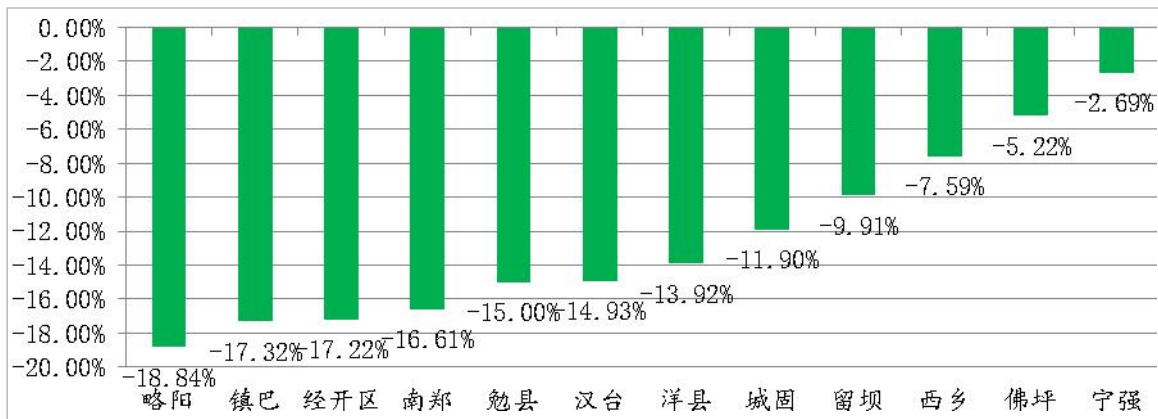
图 14 2024 年 1~4 月县（区）环境空气质量综合指数同比变化情况
