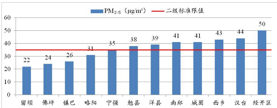
图 16 2024 年 1~4 月各县（区）PM 2.5 浓度及达标情况
