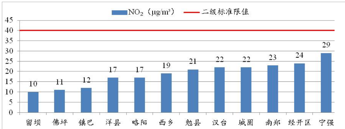
图 18 2024 年 1~4 月各县（区）NO 2 浓度及达标情况
