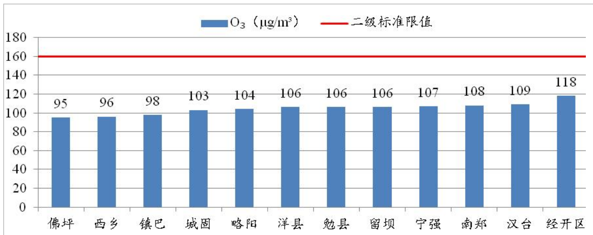
图 20 2024 年 1~4 月各县（区）O 3 浓度及达标情况
