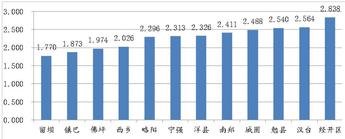
图3 2024年4月各县(区)环境空气质量综合指数
