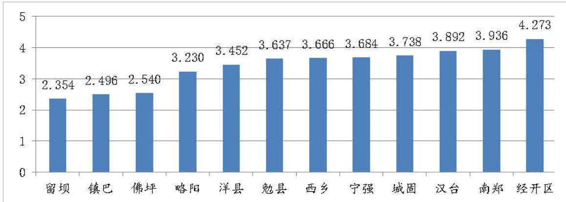
图 13 2024 年 1~4 月县（区）环境空气质量综合指数
