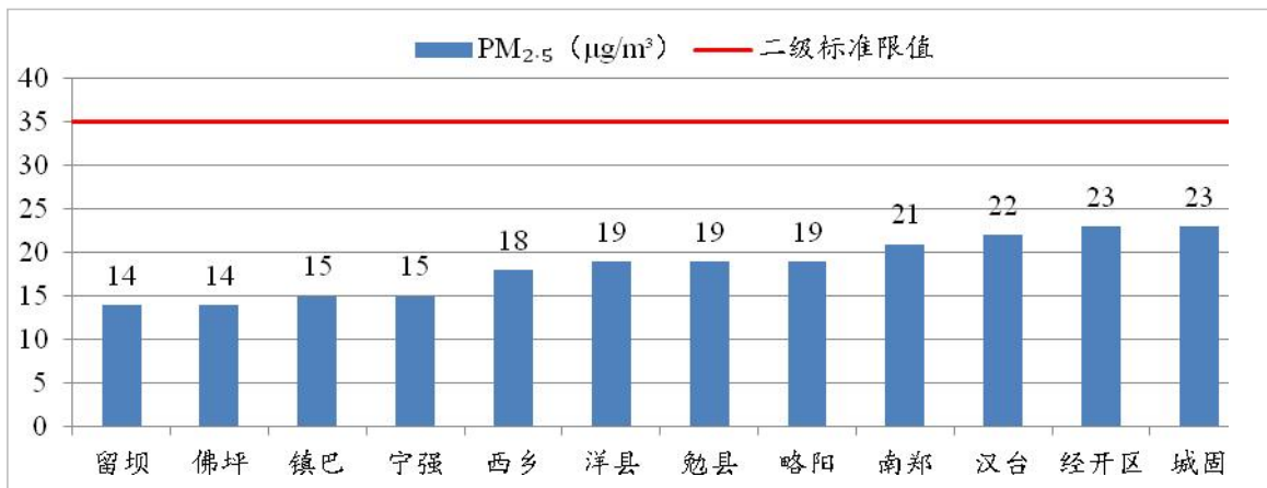
图6 2024年4月各县(区)PM 2.5 浓度及达标情况
