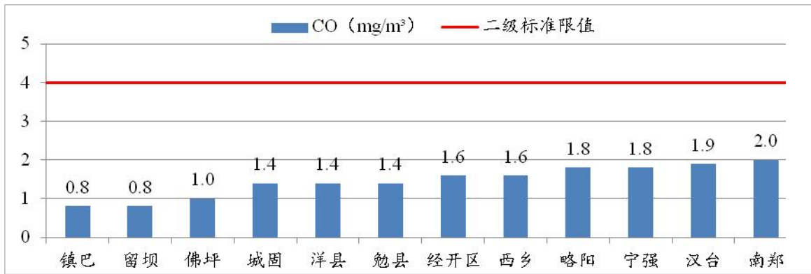
图 19 2024 年 1~4 月各县（区）CO 浓度及达标情况
