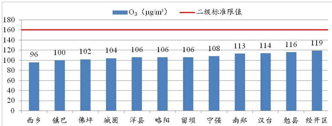
图10 2024年4月各县(区)O 3 浓度及达标情况
