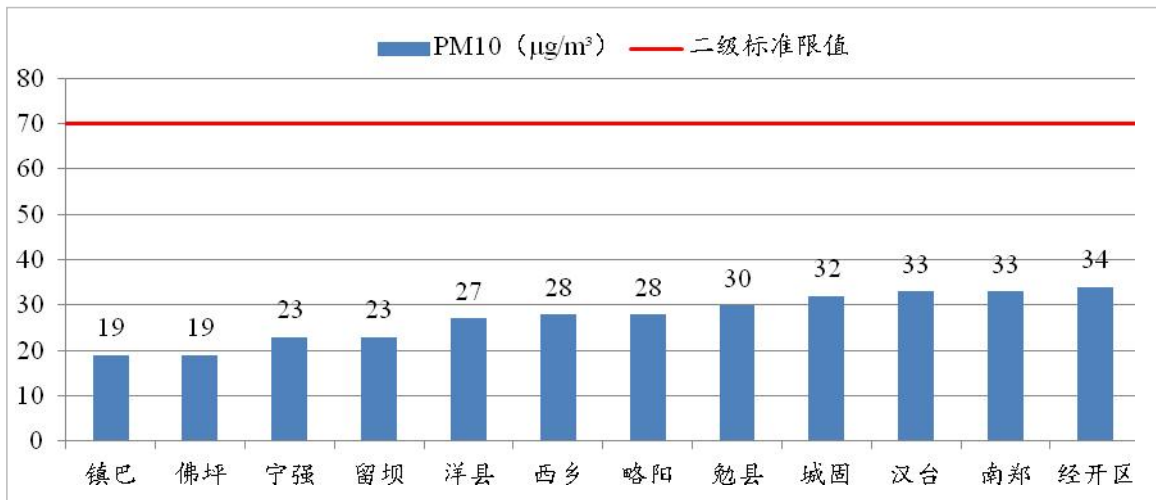
图5 2023年10月各县区pM 10 浓度及达标情况
