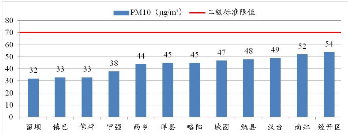
图 15 2023 年 1~10 月各县区 pM 10 浓度及达标情况
