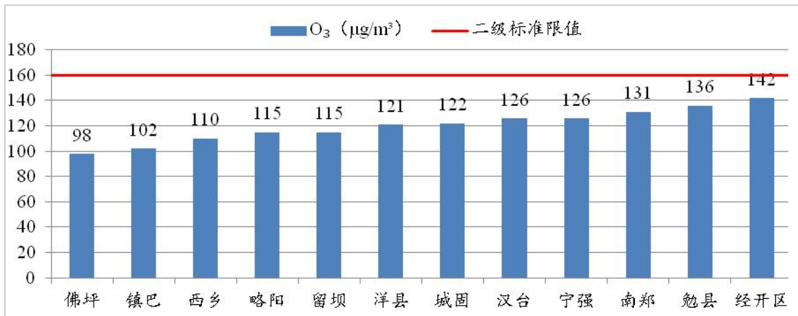
图 20 2023 年 1~10 月各县区 O 3 浓度及达标情况
