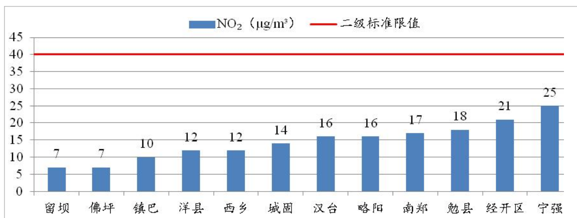
图 18 2023 年 1~10 月各县区 NO 2 浓度及达标情况
