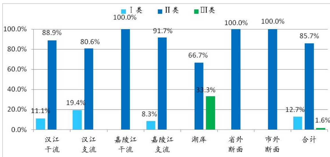
图 21 2023 年 10 月全市地表水断面水质类别比例图
