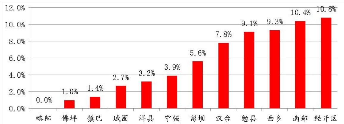
图 14 2023 年 1~10 月县区环境空气质量综合指数较去年同比变化情况
