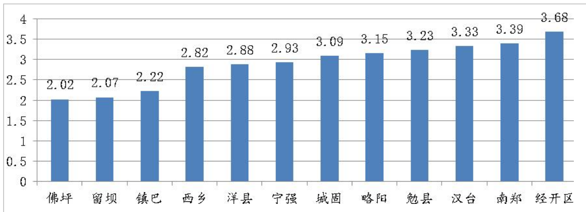
图 13 2023 年 1~10 月县区环境空气质量综合指数
