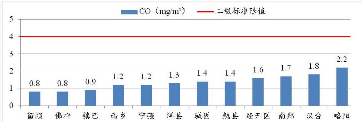
图 19 2023 年 1~10 月各县区 CO 浓度及达标情况
