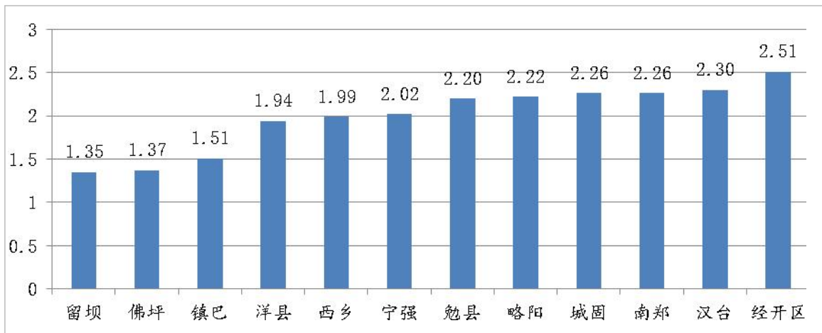
图3 2023年10月各县区环境空气质量综合指数
