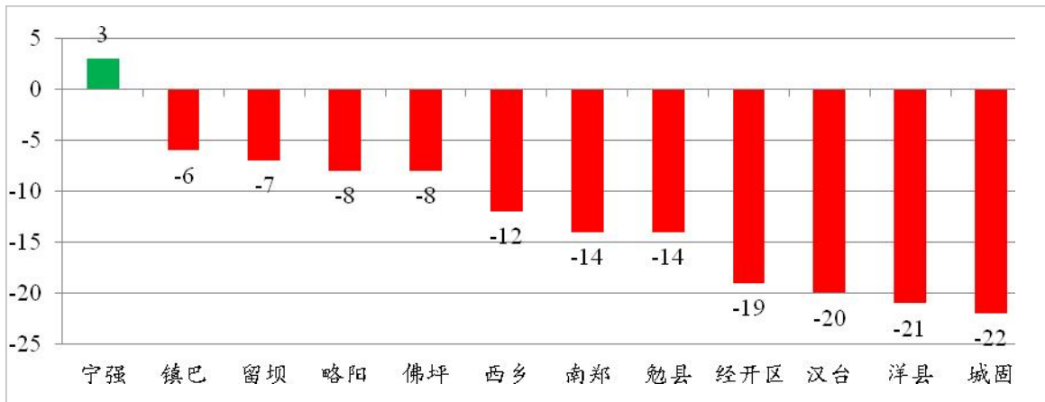
图 12 2023 年 1~10 月县区环境空气质量优良天数较去年同比变化情况 (单位: 天)
