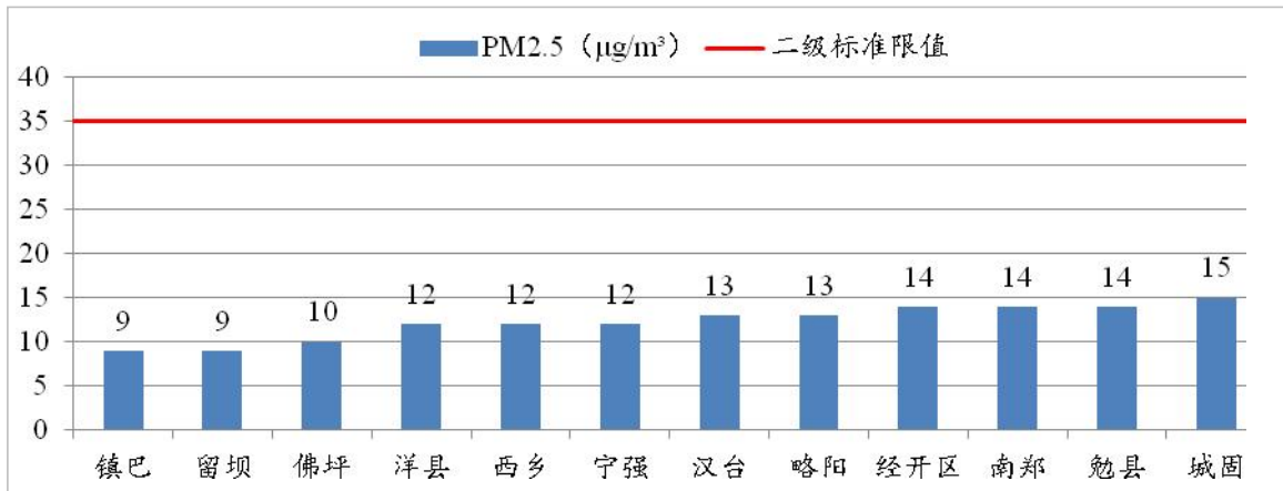
图6 2023年10月各县区pM 2.5 浓度及达标情况
