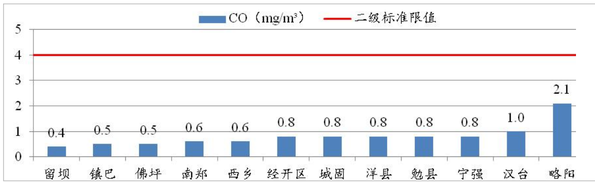
图9 2023年10月各县区CO浓度及达标情况
