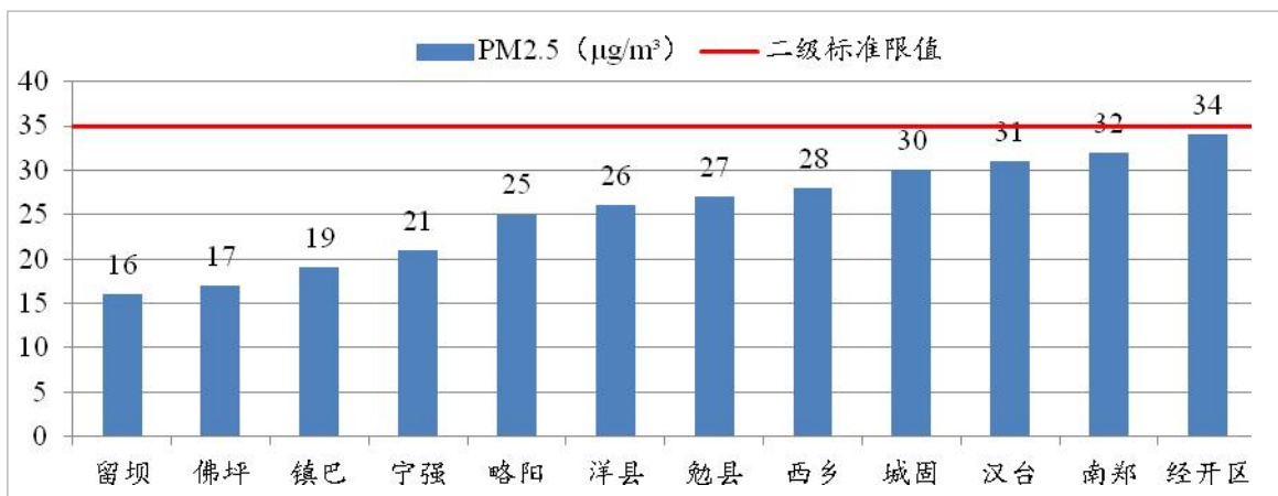
图 16 2023 年 1~10 月各县区 pM 2.5 浓度及达标情况
